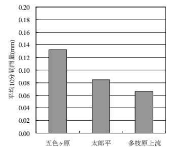
図-2 観測期間中の平均 10 分間雨量
