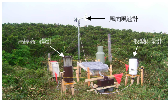
写真-1 五色ヶ原観測所の設置状況
